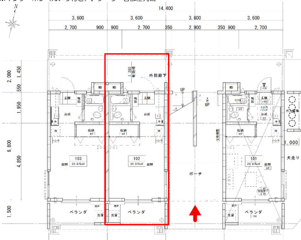
1階平面図
